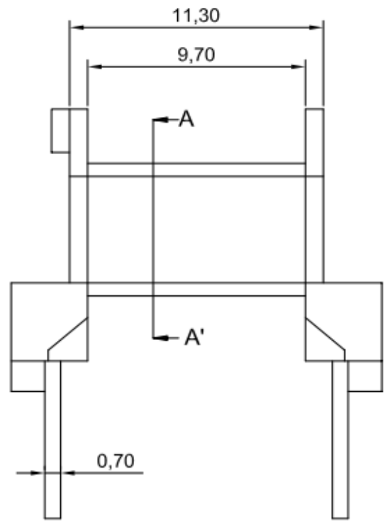
R.H.SIDE VIEW
