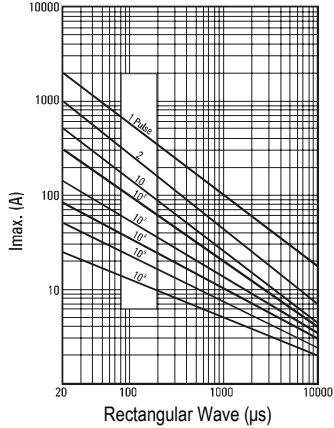
ROV14H820K – ROV14H511K
