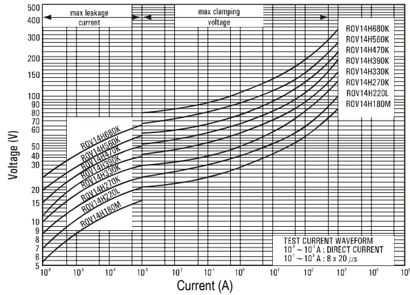
ROV14H820K – ROV14H511K
