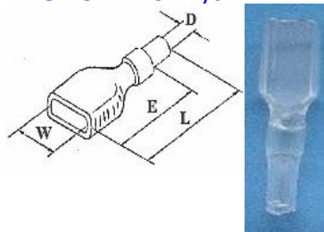
FASTON 4.8 kryt P1741H
